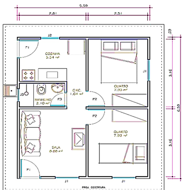
PLANTA BAIXA / LAYOUT ESCALA 1/50
