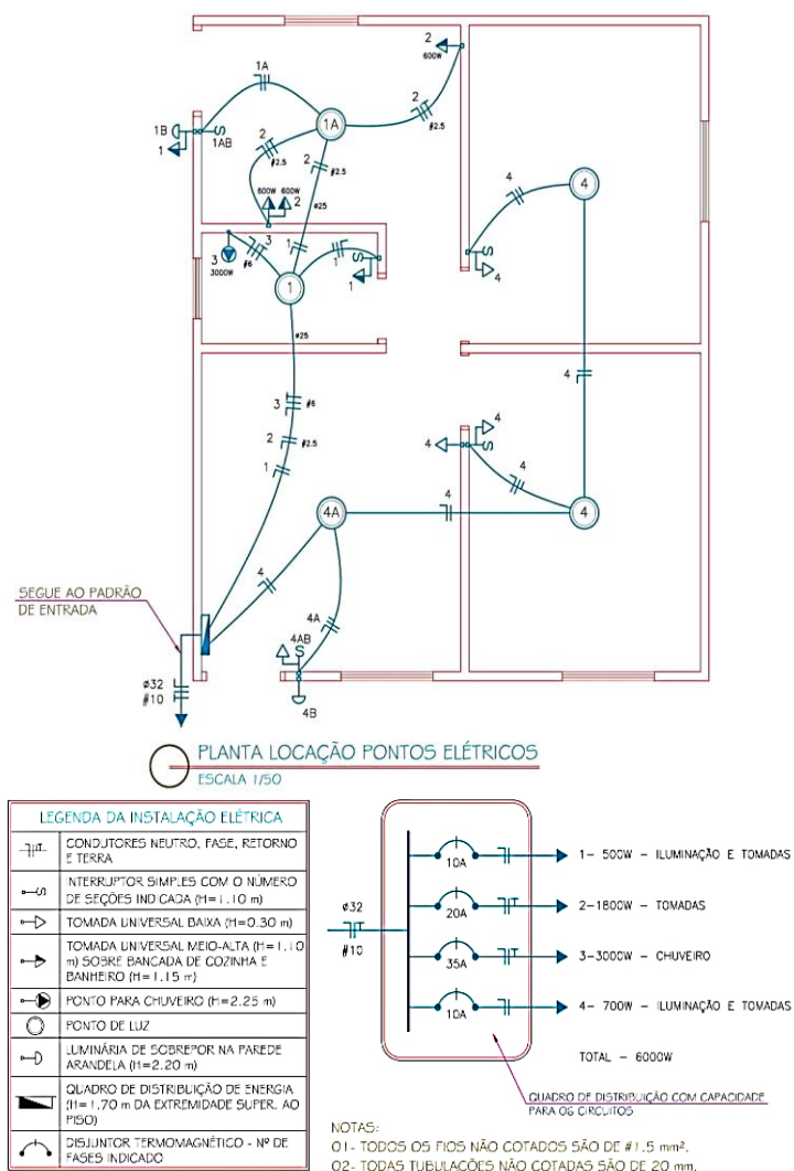
Figura 07 – Planta de Locação dos Pontos Elétricos da Residência Modelo Padrão
