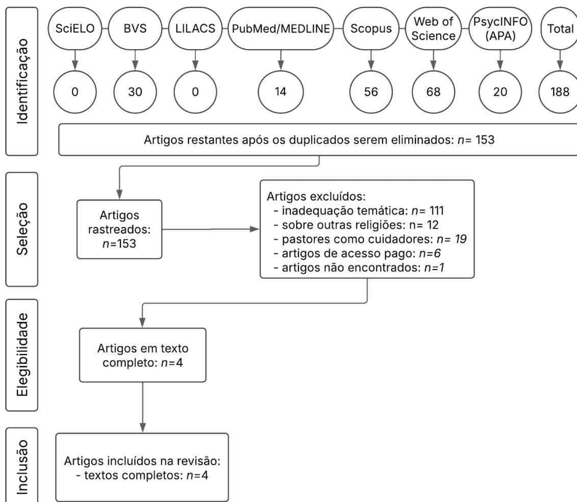
Figura 1 - Fluxograma Prisma
